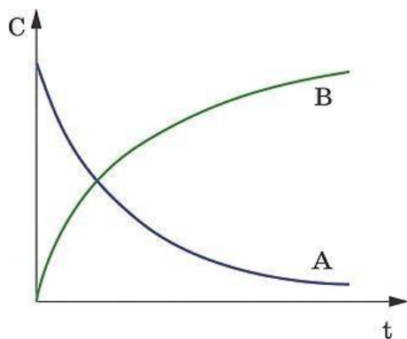
Рис. График зависимости концентрации исходных веществ и продуктов реакции от времени протекания реакции
